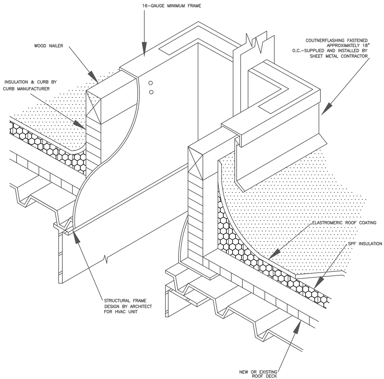
Curb_HVAC_Unit[1]
